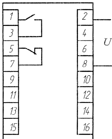
Рисунок В.1 – Схема электрическая подключения реле РН -53, РН-54 (вид спереди).
